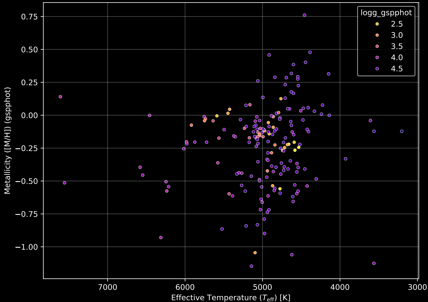
APOGEE DR17 Field: [K2_C8_122-57_btx] Stellar Population Parameters (n= 181)
